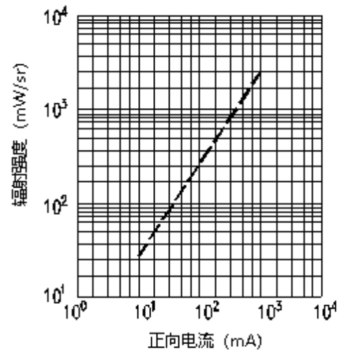
图四：相对强度和正向电流关系曲线
