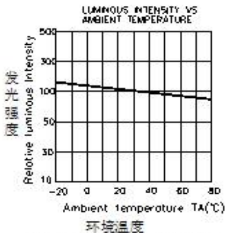
发光强度与环境温度关系
