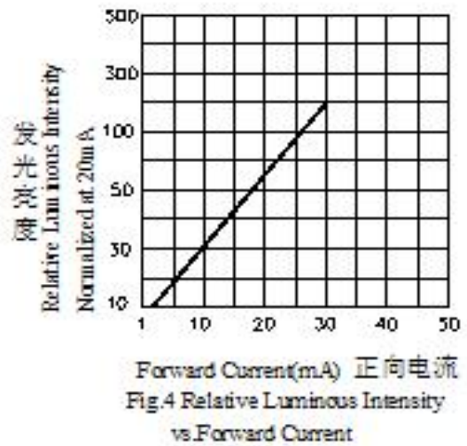
正向电流与发光强度关系
