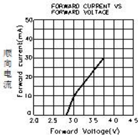
正向电压
