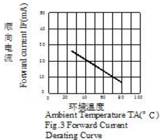
电流与环境温度关系
