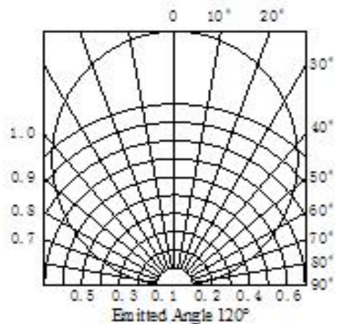
成品发光角度
