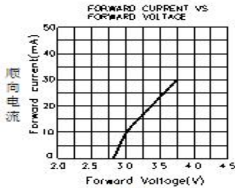
正向电压
