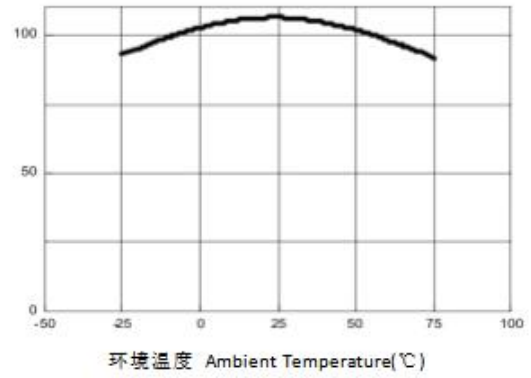
输出特性
